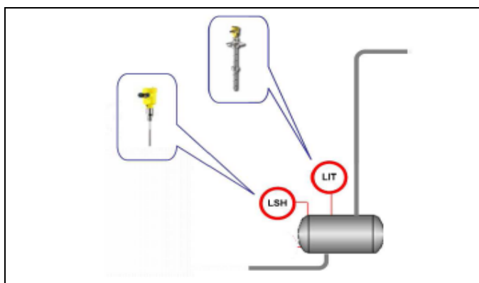
Figura 4 – Instrumentación de tanques diarios
