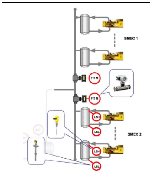
Figura 5 – Instrumentación de grupos SMEC
