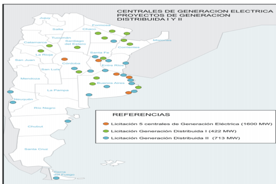
Figura 1 – Centrales térmicas de los proyectos de generación distribuída I y II (Información suministrada por la empresa ENARSA)
