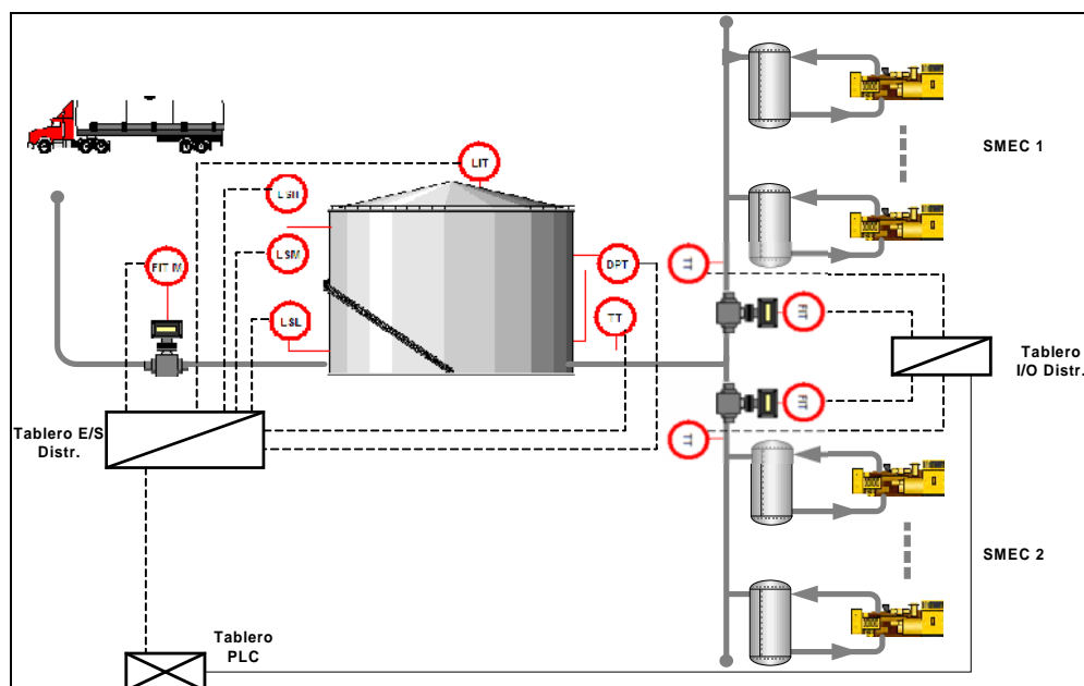
Figura 2 – Arquitectura del SMC de gas-oil
