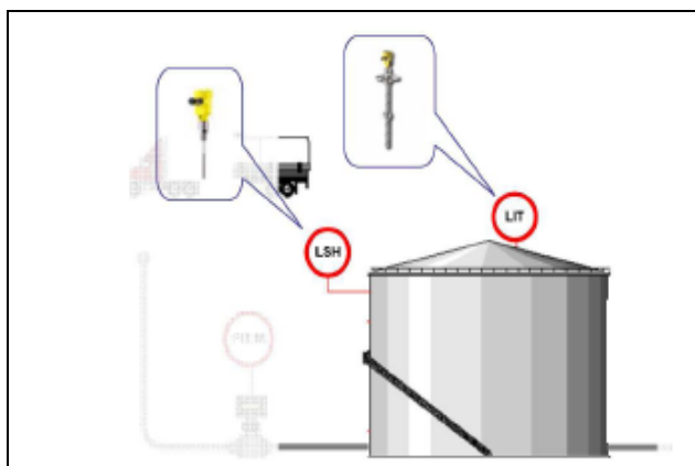
Figura 3 – Instrumentación de tanques principales
